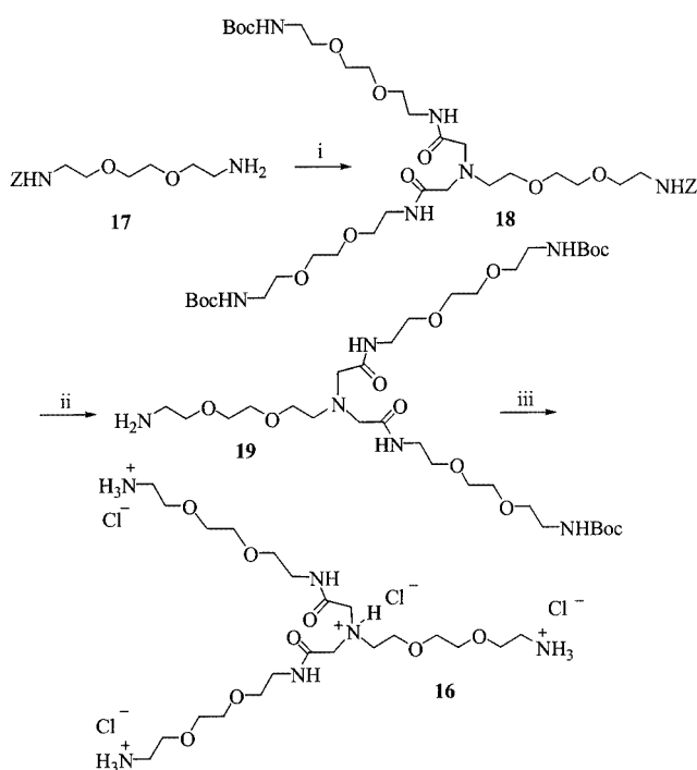
Scheme 4. i: 13 , TEA, \text{CH}_2\text{Cl}_2 ; ii: \text{H}_2 , Pd/C, methanol; iii: HCl, methanol
