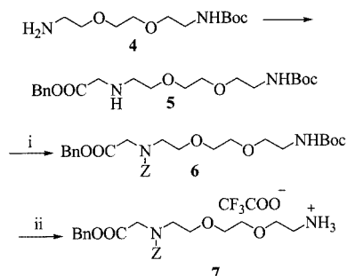
Scheme 1. i: ZCl, DCM; ii: TFA, DCM
